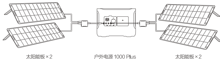
太阳能板 × 2
